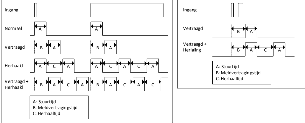
Figuur 1: Schematische weergaven ingangenfunctie
