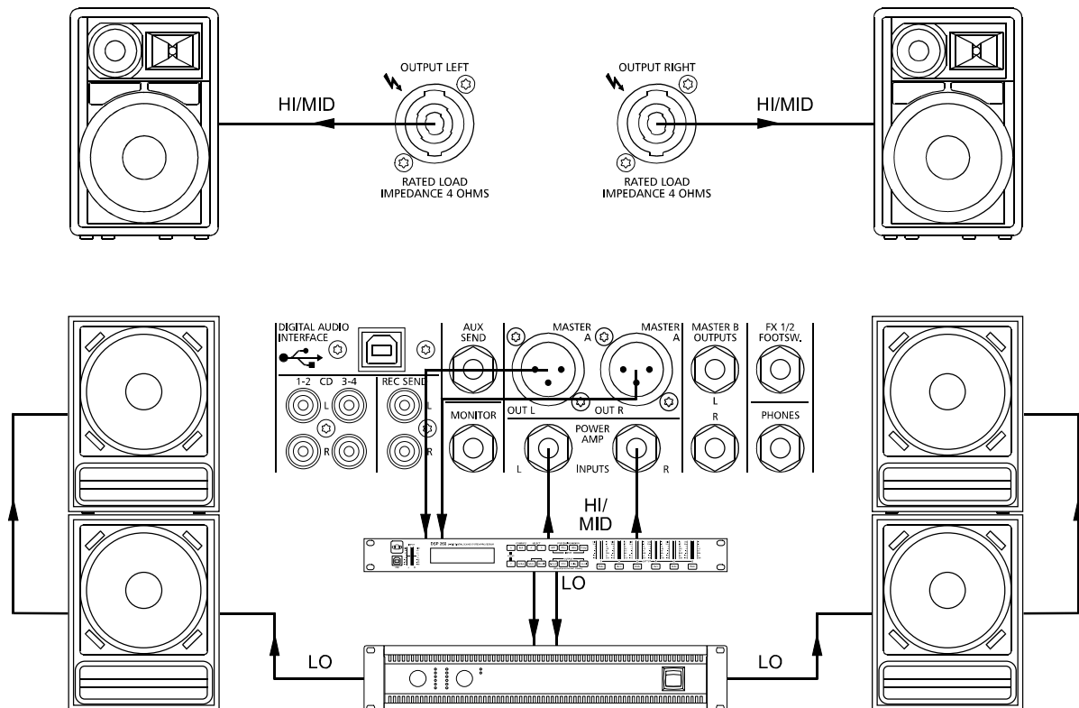
Abbildung 6-5: Aktiv Stereo 2-Weg System
